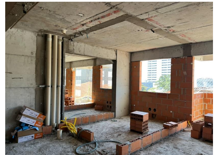
Alvenaria/ Fechamento – 8º Pav
