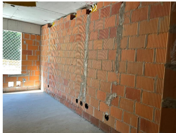
Embutidos em Alvenaria – 2º Pav
