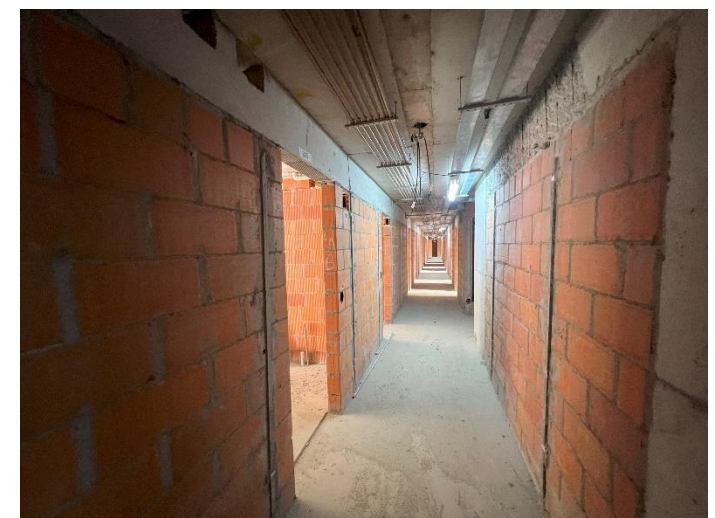
Eletrocalhas – 2º Pav
