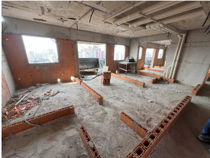
Marcação de Alvenaria – 17º Pav
