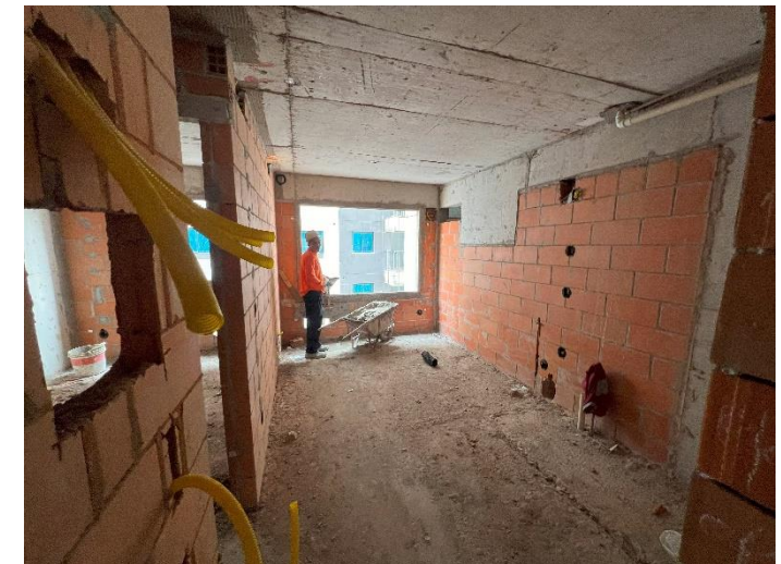
Embutidos em Alvenaria – 9º Pav
