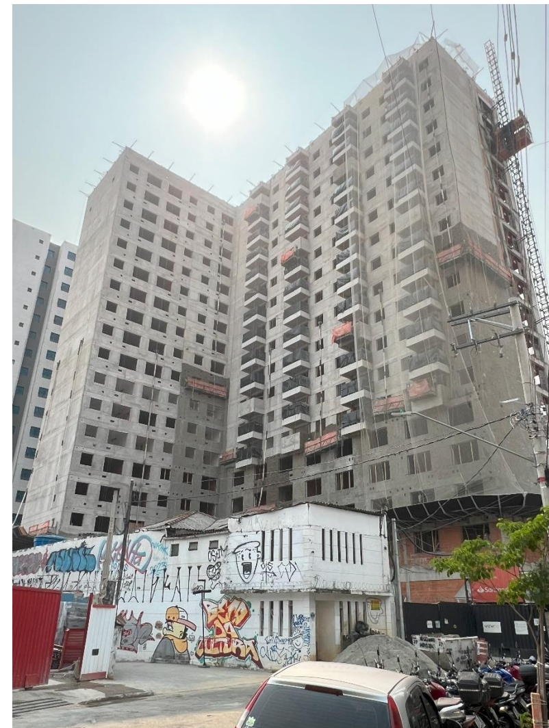
Reboco da Fachada – Foto dia 02/Set/2024
